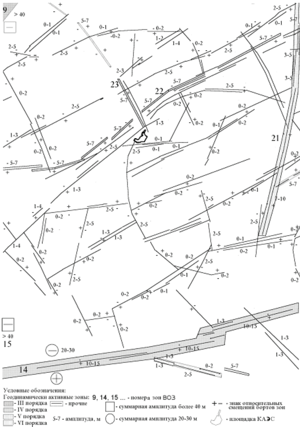
Рис. 3. Результаты уточнения геодинамических условий ближнего района размещения Калининской АЭС. Фрагмент схемы геодинамически активных зон ближнего района размещения Калининской АЭС.
