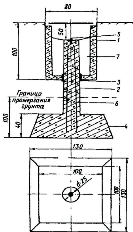
Рис. 3. Репер с бетонным монолитом
