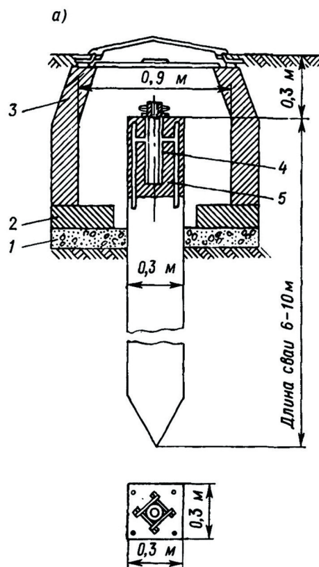
Рис. 4. Свайный репер
