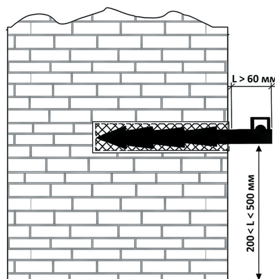
Рис. 2. Стенная марка
