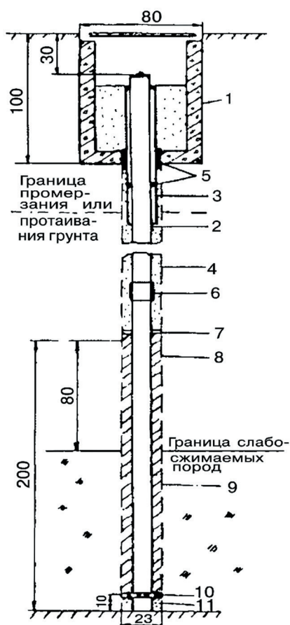
Рис. 2. Трубчатый глубинный репер
