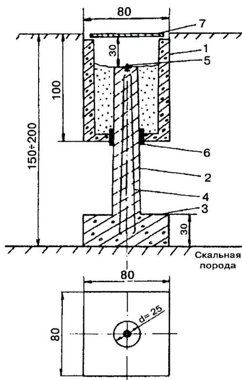
Рис. 1. Репер для скальных грунтов
